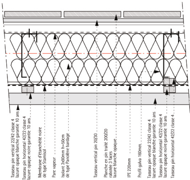
COUPE 1/10°
